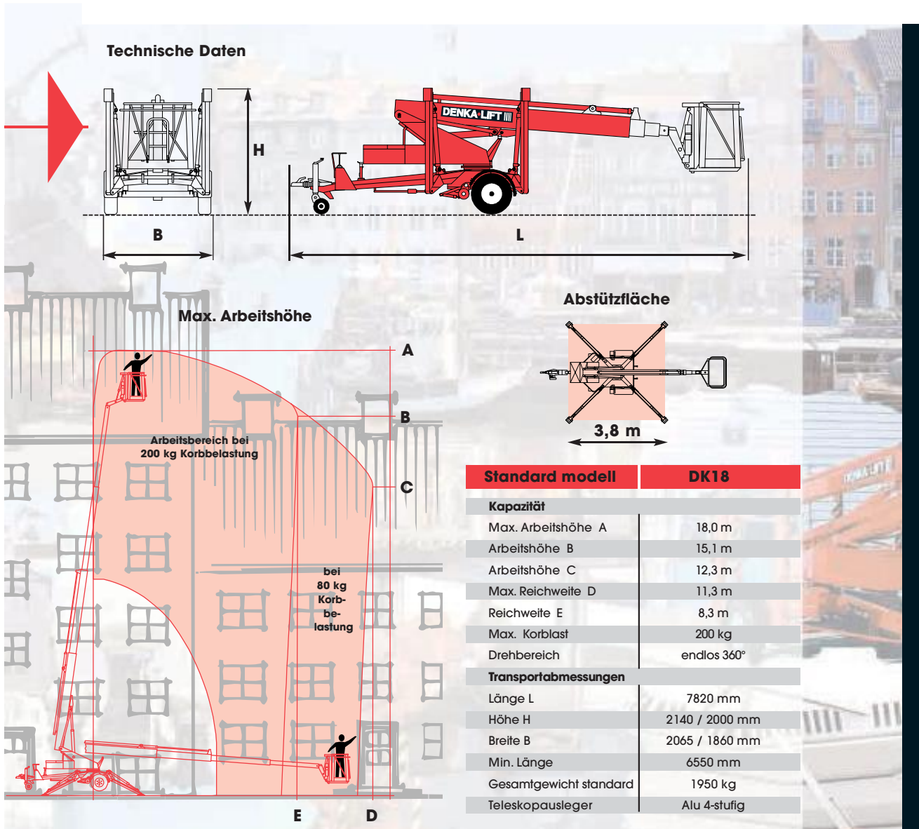
Anhänger - Arbeitsbühne Teleskop - Anhänger AT18
